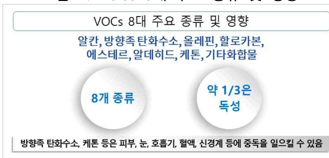
<그림1 : VOCs 8대 주요 종류 및 영향>
